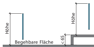
Abb. 2: Höhe Schutzelement
