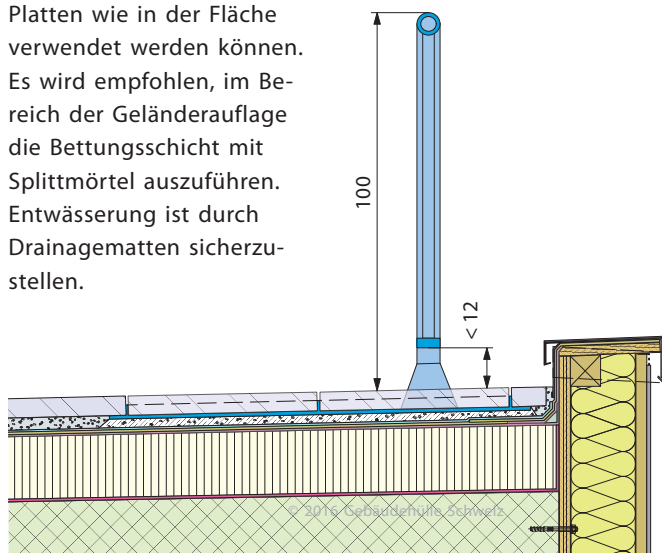
Abb. 19: Systemgeländer mit Auflast der Nuttschicht. Systemanforderungen beachten
